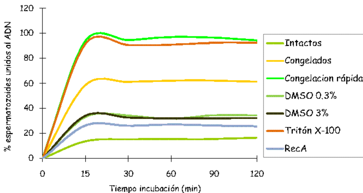
FIGURA 54. Cinética de unión entre el transgén y los espermatozoides sometidos a diferentes tratamientos a lo largo del tiempo de incubación (0, 15, 30, 60, 90 y 120 min).
