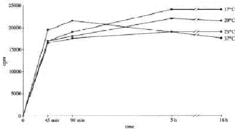
FIGURA 8. Optimización de la temperatura de incubación ADN/espermatozoide del protocolo de SMGT.
